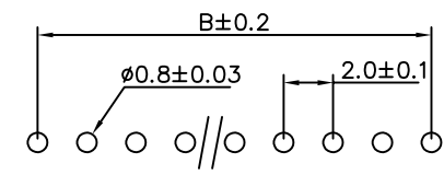
P.C.B LAYOUT
